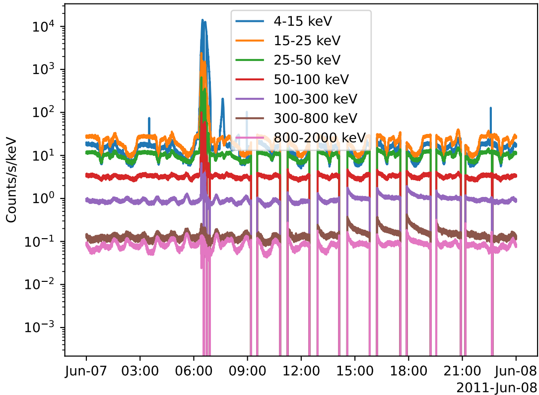
Fermi GBM Summary data ['NAI_05']
